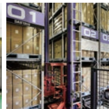
自動物流倉庫内部
